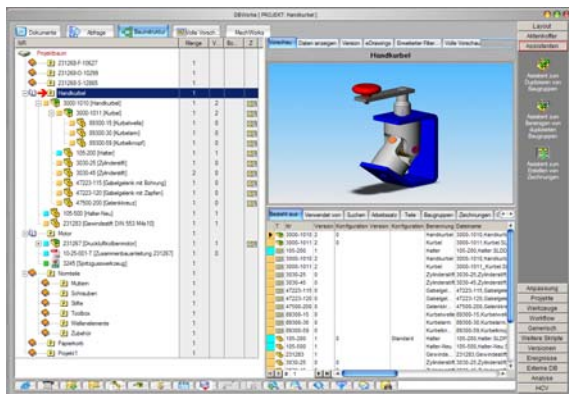
DBWorks Browser
